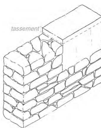
Figure 10: Soubassement* en escalier avec bauge pour récupérer les niveaux, en attente de tassement*
