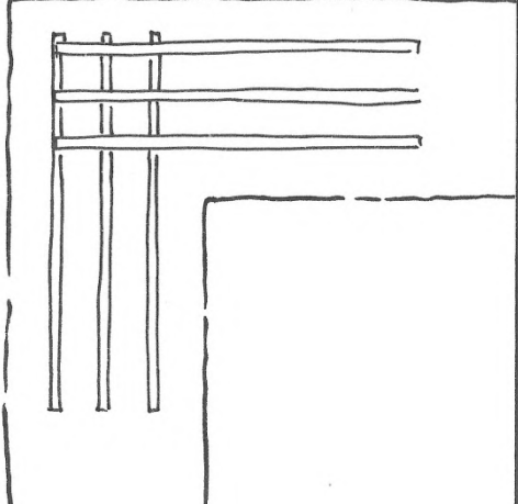
Figure 25: Agrafe* en noisetier, roseau, bambou ou osier
